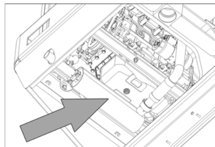
1 Паливний кран 2 Паливний фільтр → Закрити паливний кран. → Відгвинтити та замінити паливний фільтр.
