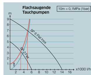
Kennlinie 1"-PrimoFlex®-Schlauch ..... Verschobene Kennlinie 1 1/4"-PrimoFlex®-Schlauch
