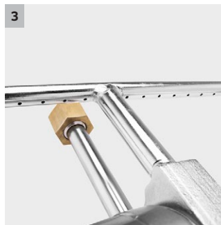
3 Beépített permetezőrúd
