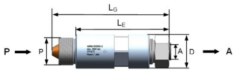
Обратный клапан RV 3000-E
