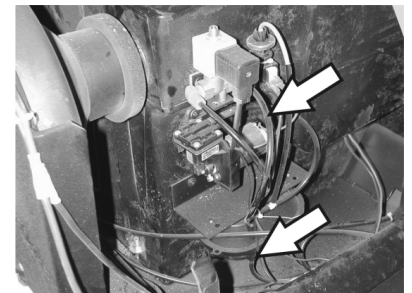
Alipainepumpun ja alipainerasian letkuliitäntä (varaaja)
