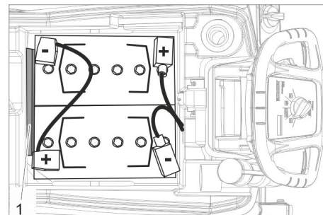
Batterie 6.654-093.0 1 Entretoises
