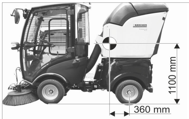
Poloha ťažiska pri plne naloženom prístroji.
