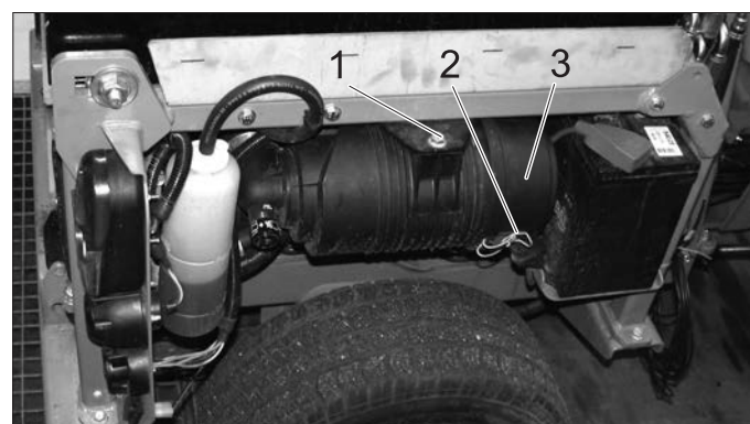
1 Винт 2 Скоба 3 Корпус на въздушния филтър
