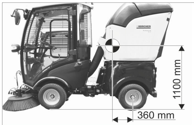
Těžiště při plně naloženém přístroji.
