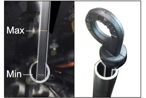
Resim: Benzinli motorlarda yağ seviyesinin ölçülmesi (KM 105/... ve KM 125/...)
