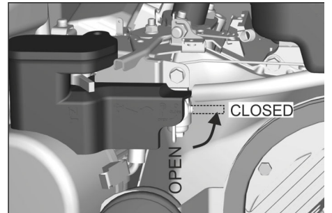
Εικόνα: Κλείσιμο στρόφιγγας καυσίμου (βενζινοκινητήρας)
