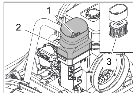
Bilde: Bensinmotor (KM 105/...)
