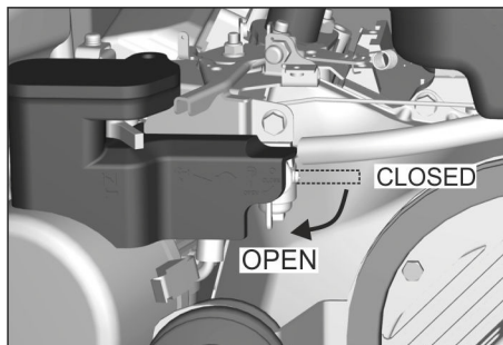
Bild: Öppna bränslekranen (bensin-/gasmotor)
