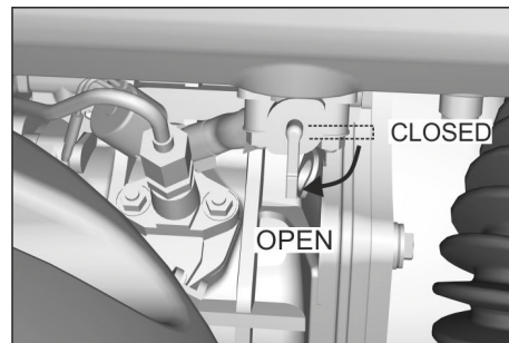
Abbildung: Kraftstoffhahn öffnen (Dieselmotor)
