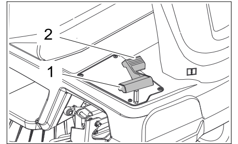
Şekil: Yakıt musluğunun açılması (benzinli/gazlı motor)
