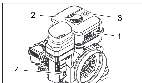
Figura: Motor a gasolina (KM 105/...)
