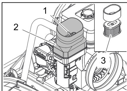
Abbildung: Benzinmotor (KM 105/...)
