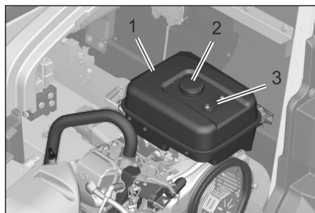
Figure : Moteur thermique (KM 125/...)
