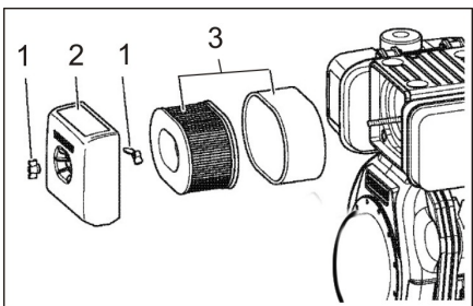
Resim: Benzinli motor (KM 105/...)
