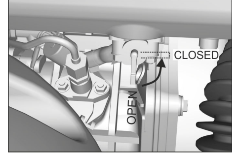
Şekil: Yakıt musluğunun kapatılması (dizel motor)
