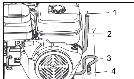
Abbildung: Benzinmotor (KM 105/...)
