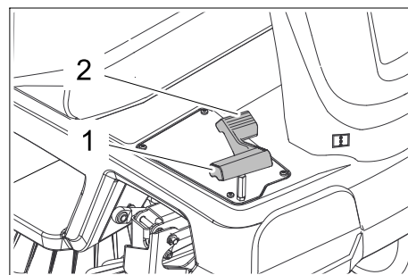
Bild: Öppna bränslekranen (bensin-/gasmotor)
