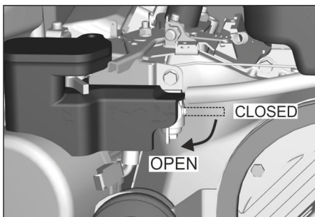
Figur: Åbning af brændstofhane (benzin/gasmotor)
