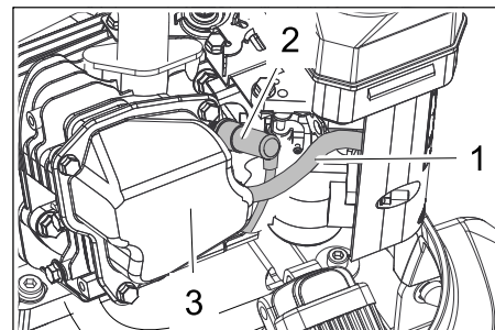
Figura: motor de gasolina (KM 105/...)
