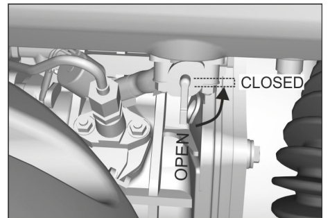
Εικόνα: Κλείσιμο στρόφιγγας καυσίμου (πετρελαιοκινητήρας)
