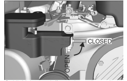
Şekil: Yakıt musluğunun kapatılması (benzinli motor)
