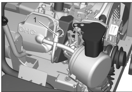
Kuva: Bensinimoottori (KM 125/...)
