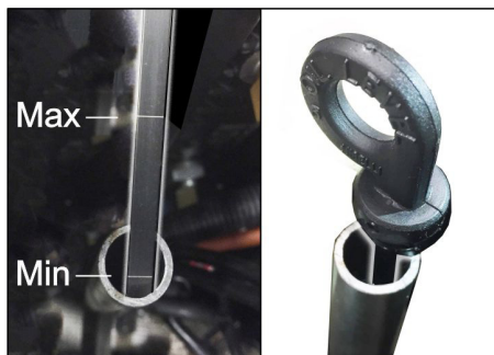
Bilde: Måle oljenivået i bensinmotorer (KM 105/... og KM 125/...)
