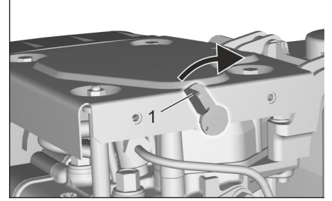
Şekil: Dekompresyon kolu (dizel motor)
