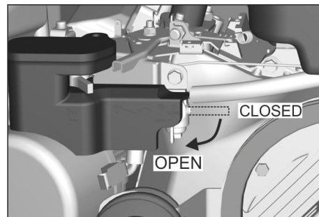
Εικόνα: Άνοιγμα στρόφιγγας καυσίμου (κινητήρας βενζίνης/αερίου)
