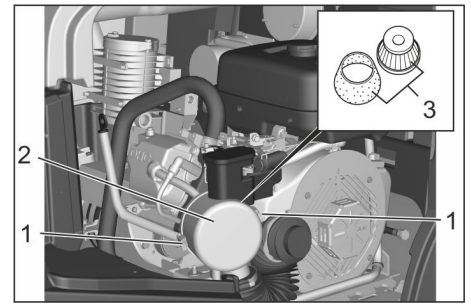
Figure: Petrol motor (KM 125/...)
