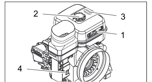
Resim: Benzinli motor (KM 105/...)
