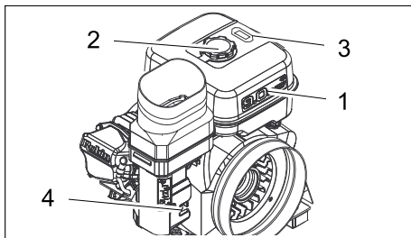
Σχήμα: Βενζινοκινητήρας (KM 105/...)
