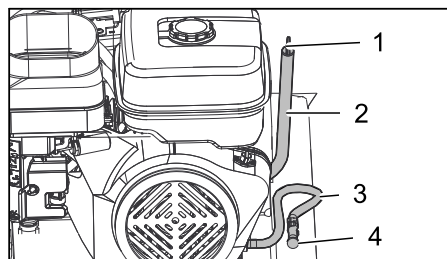
Figura: motor de gasolina (KM 105/...)
