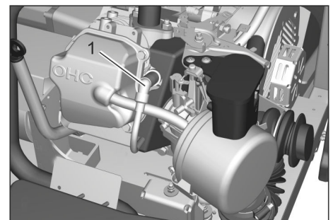
Figure: Petrol motor (KM 125/...)
