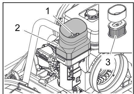
Figure : Moteur thermique (KM 105/...)
