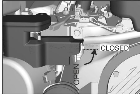
Kuva: Sulje polttoainehana (bensiniinmoottori)
