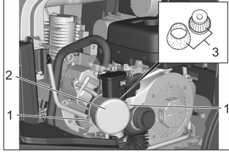
Resim: Benzinli motor (KM 125/...)
