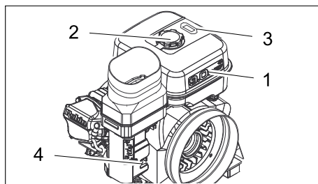
Figura: motor de gasolina (KM 105/...)
