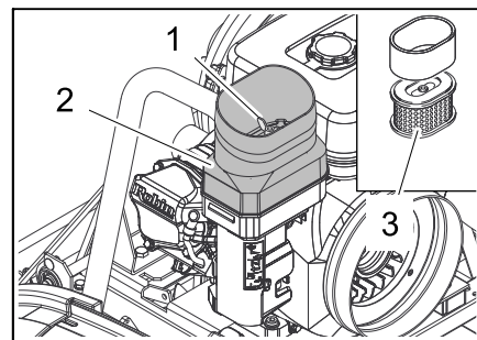
Kuva: Bensiniinimoottori (KM 105/...)
