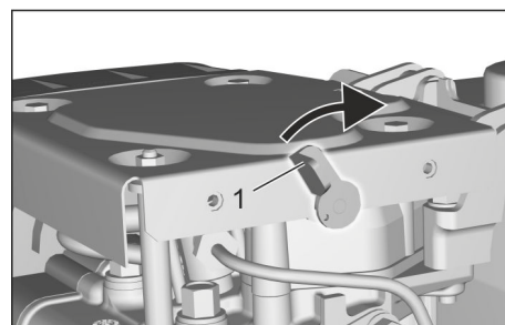
Figure : Levier de décompression (moteur diesel)
