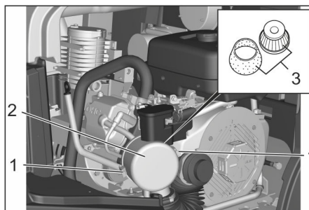
Σχήμα: Βενζινοκινητήρας (KM 125/...)
