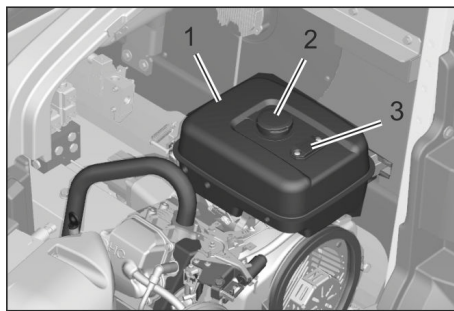
Bilde: Bensinmotor (KM 125/...)
