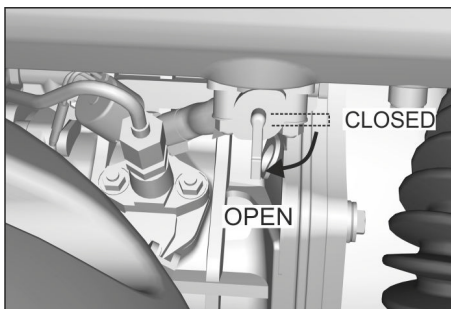
Figur: Åbning af brændstofhanen (dieselmotor)
