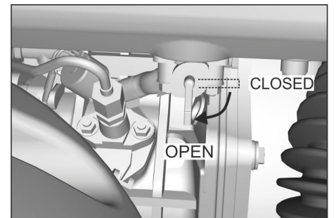
Bilde: Åpne drivstoffkranen (dieselmotor)
