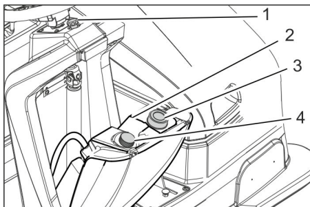
Bild: Främre hydrauliktank
