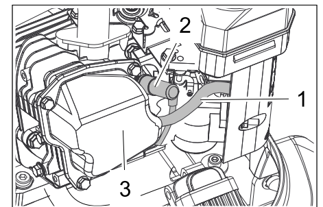
Figure: Petrol motor (KM 105/...)
