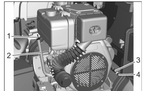
Εικόνα: Ντιζελοκινητήρας (KM 125/...)
