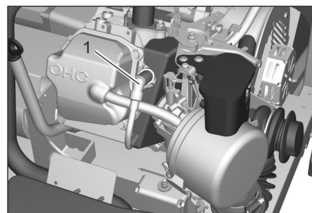
Σχήμα: Βενζινοκινητήρας (KM 125/...)
