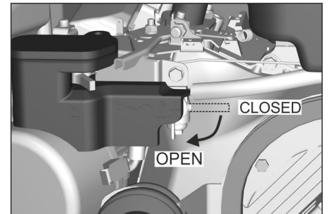
Bilde: Åpne drivstofftilførselen (bensin-/gassmotor)
