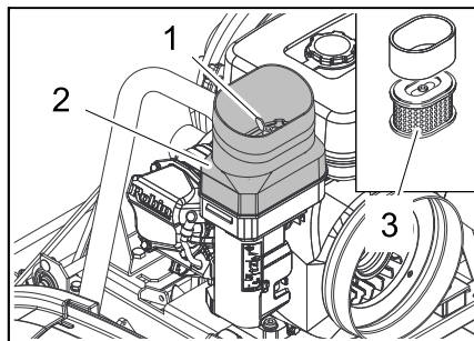
Σχήμα: Βενζινοκινητήρας (KM 105/...)
