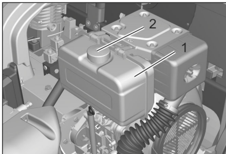
Figure: Dieselmotor (KM 125/...)
