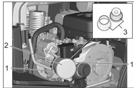
Figur: Benzinmotor (KM 125/...)
