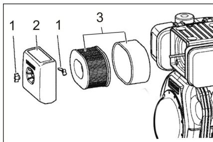
Imagen: motor diesel (KM 125/...)
