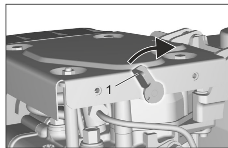
Figura: Leva di decompressione (motore diesel)
