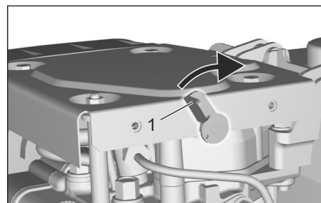
Abbildung: Dekompressionshebel (Dieselmotor)
