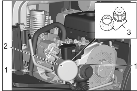
Figura: motor de gasolina (KM 125/...)
