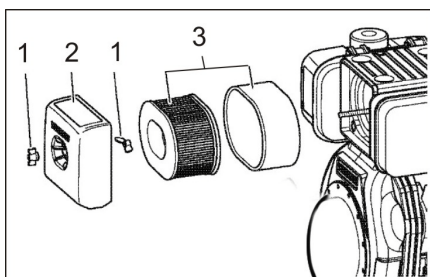
Abbildung: Benzinmotor (KM 105/...)
