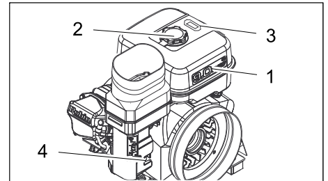
Kuva: Bensiinimoottori (KM 105/...)
