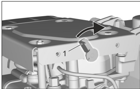
Εικόνα: Μοχλός αποσυμπίεσης (πετρελαιοκινητήρας)
