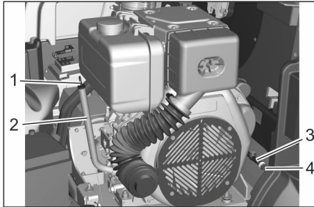
Kuva: Dieselmoottori (KM 125/...)
