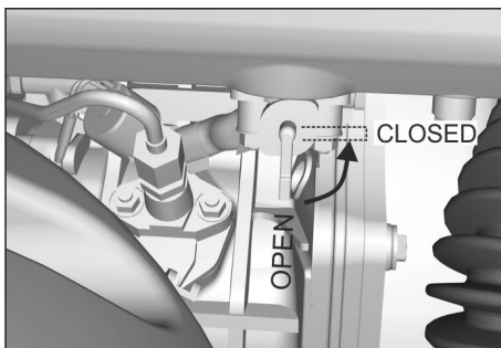
Figur: Lukning af brændstofhane (dieselmotor)
