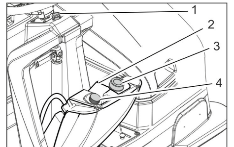
Abbildung: Vorderer Hydrauliktank
