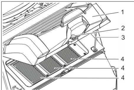
Abbildung: KM 125/... mit 3 Flachfaltenfil-ter; KM 105/... besitzt 2 Flachfaltenfilter
