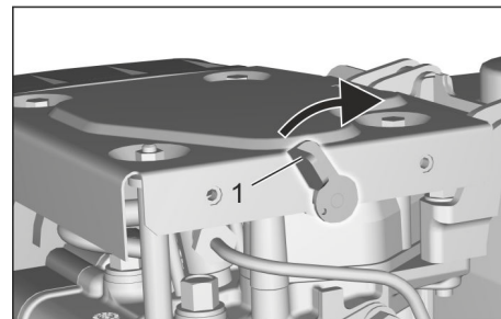
Imagen: palanca de descompresión (motor diesel)
