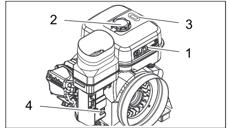
Figure: Petrol motor (KM 105/...)
