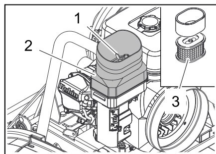
Figur: Benzinmotor (KM 105/...)
