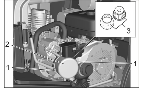
Bild: Bensinmotor (KM 125/...)
