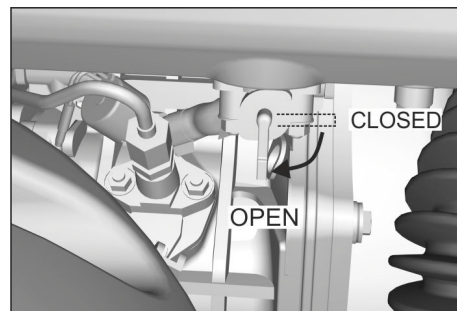
Εικόνα: Άνοιγμα στρόφιγγας καυσίμου (πετρέλαιοκινητήρας)
