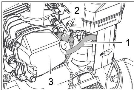
Afbeelding: Benzinemotor (KM 105/...)
