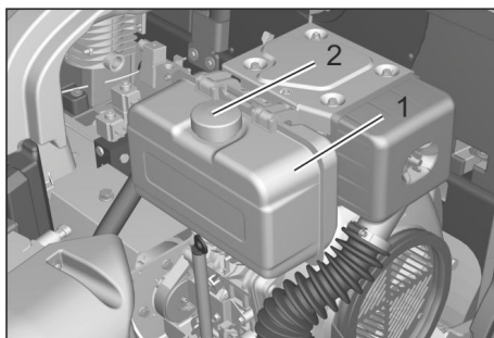
εικόνα: Ντιζελοκινητήρας (KM 125/...)
