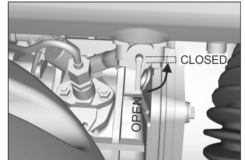
Abbildung: Kraftstoffhahn schließen (Dieselmotor)
