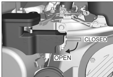
Afbeelding: Brandstofkraan openen (benzine-/gasmotor)
