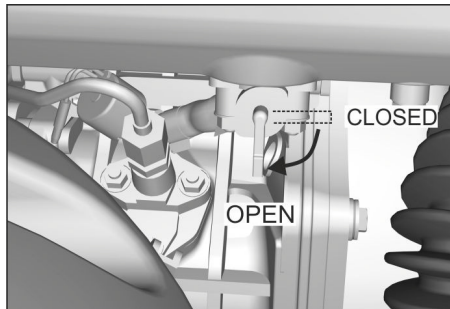
Şekil: Yakıt musluğunun açılması (dizel motor)
