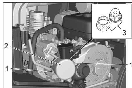
Bilde: Bensinmotor (KM 125/...)
