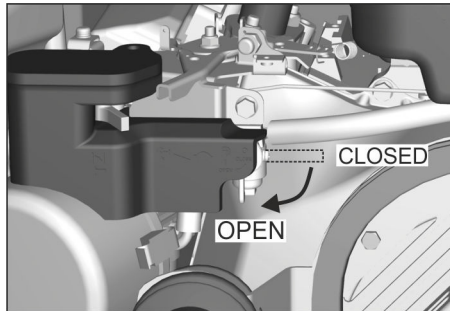
Şekil: Yakıt musluğunun açılması (benzinli/gazlı motor)
