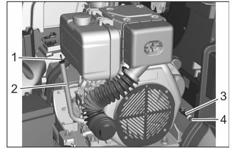
Şekil: Dizel motor (KM 125/...)
