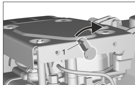
Bild: Dekompressionsspak (dieselmotor)
