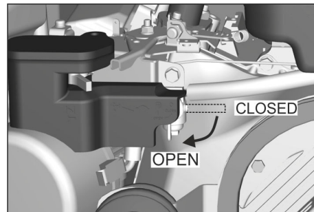
Abbildung: Kraftstoffhahn öffnen (Benzin-/Gasmotor)
