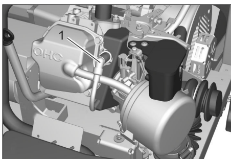
Afbeelding: Benzinemotor (KM 125/...)
