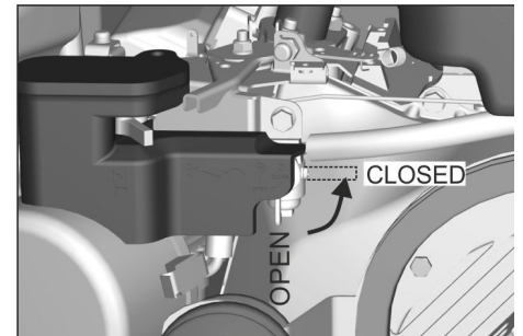
Abbildung: Kraftstoffhahn schließen (Benzinmotor)
