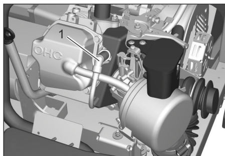
Figura: Motor a gasolina (KM 125/...)
