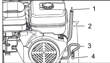
Resim: Benzinli motor (KM 105/...)
