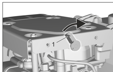
Kuva: Dekompressiovipu (dieselmoottori)
