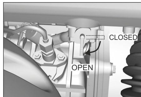
Afbeelding: Brandstofkraan openen (dieselmotor)
