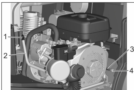
Figur: Benzinmotor (KM 125/...)
