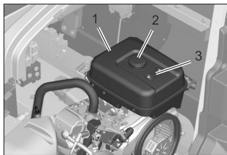
Σχήμα: Βενζινοκινητήρας (KM 125/...)
