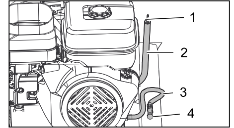
Σχήμα: Βενζινοκινητήρας (KM 105/...)
