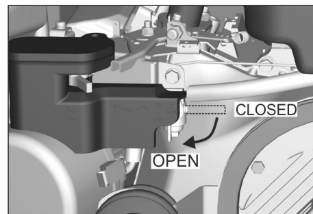
Imagen: abrir el grifo de combustible (motor de gasolina/gas)
