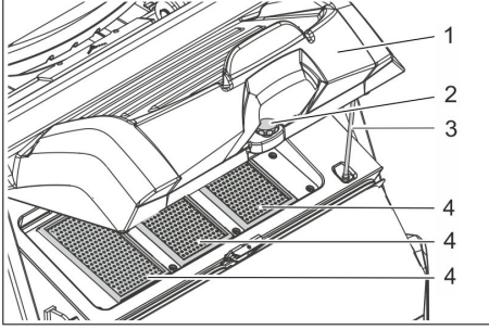
Şekil: 3 yassı katlama filtrelili KM 125/...; KM 105/..., 2 yassı katlama filtresine sahiptir
