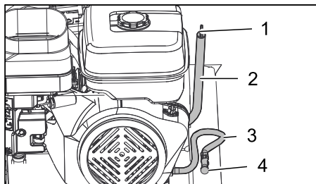
Bilde: Bensinmotor (KM 105/...)
