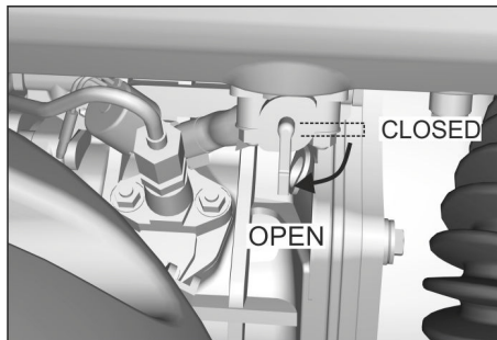
Bild: Öppna bränslekranen (dieselmotor)
