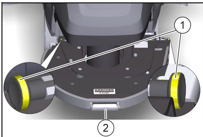
① Boulon d'arrêt de tige de poussée
