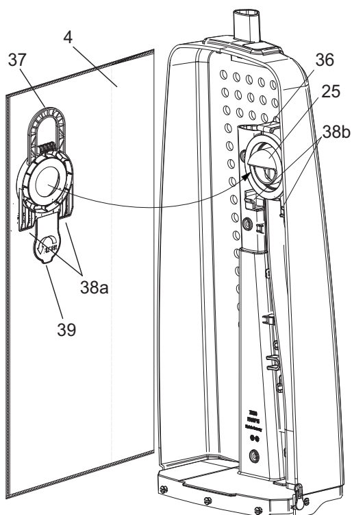
Couvercle du sac filtrant non illustré
