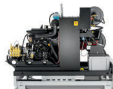
Skid 設置モデル
