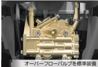
オーバーフローバルブを標準装備
