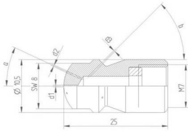
Форсунка для очистки труб 10
