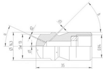
Форсунка для очистки труб 14
