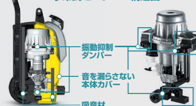
水冷式モーター＜構造図＞
