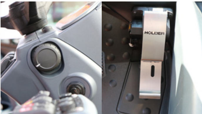
Motordrehzahl elektronisch vorwählbar mit Memory-Funktion / feinfühliges elektronisches Fußpedal
