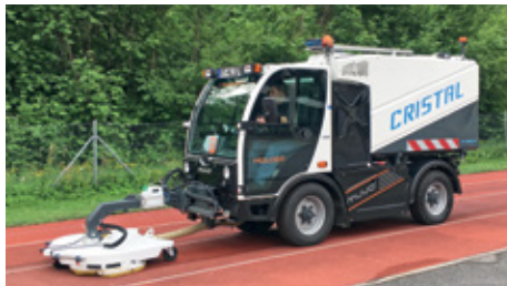
MUVO mit Hochdruckreinigungsanlage
