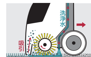
カーペット洗浄機洗浄イメージ 洗浄水を吹き付け、パキュム機能で汚れと洗浄水を同時に吸い取ります。
