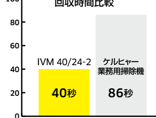
ショットブラスト約9kgの回収時間比較
