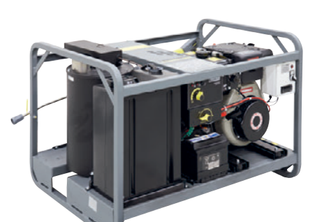
6. HDS 1000 DE WEED (エンジンモデル)
