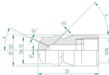
Rohrreinigungsdüse 14 Anzugsdrehmoment 20-30 Nm (14,5-22 ft-lb)
