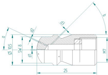
Rohrreinigungsdüse 10 Anzugsdrehmoment 10-15 Nm (7,5-11 ft-lb)
