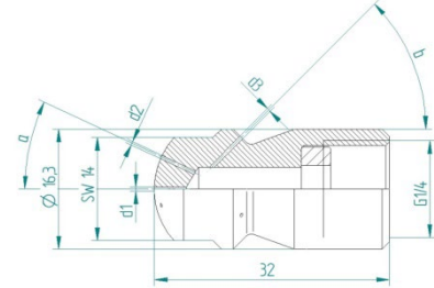
Rohrreinigungsdüse 16 Anzugsdrehmoment 40-50 Nm (29,5-35 ft-lb)
