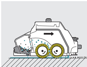
除塵機能【ブレスイープ】 ローラーブラシの特徴として、ゴミコンテナを別途設けることで、大きなゴミはブラシの回転によりコンテナで回収することができます。除塵の人工を削減しつつ、小石といった床を傷つける恐れのある物も回収できます。
